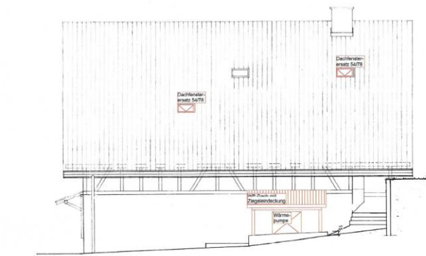
Nordostfassade
